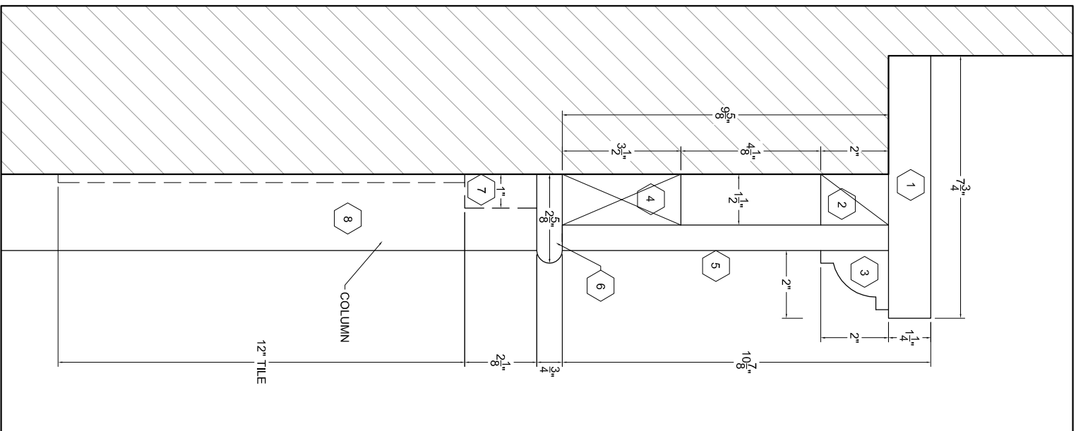
DETAIL A SCALE: 3"=1'
